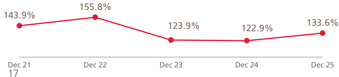
LCR (%)
