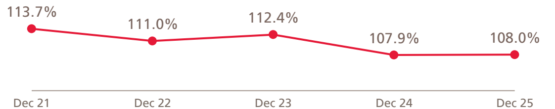
NSFR (%)
